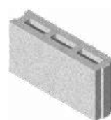
L x B x H in cm: 49,7 x 11,5 x 24,8 8 DF HPL/N+F
